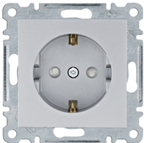
Розетка з з/к з захистом контакті в Lumina, срібна, 16A/230В
